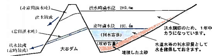
大谷ダム 貯水池断面図
